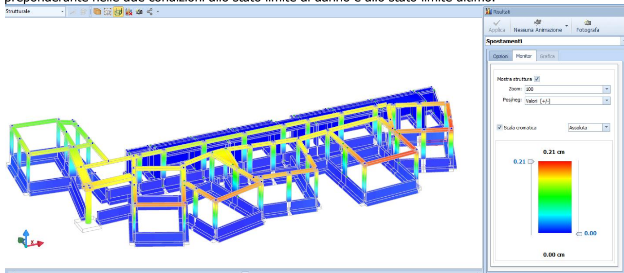
Spostamenti allo stato limite di danno per sisma in direzione X
