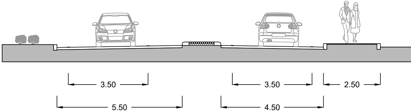
Sezione C-C
