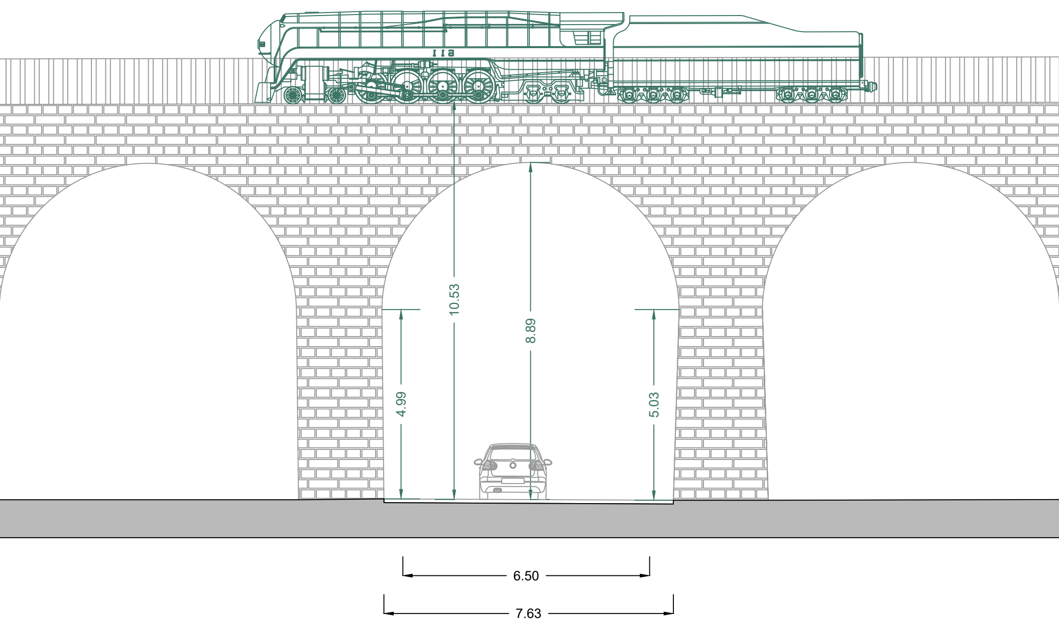
Sezione G-G
