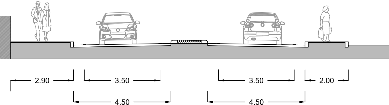
Sezione E-E
