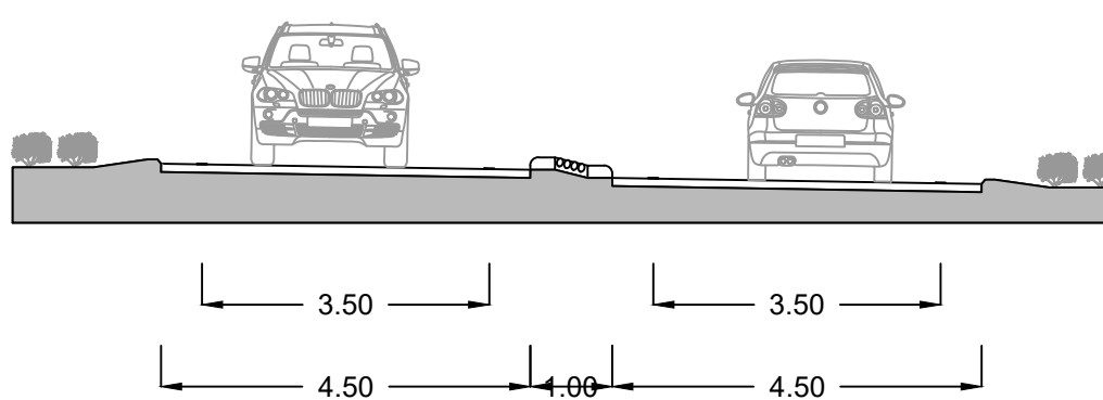
Sezione A-A
