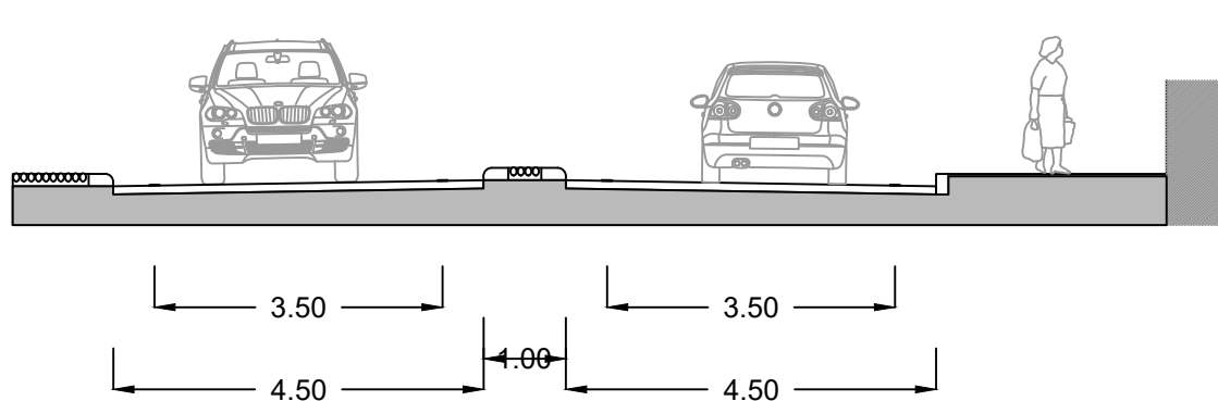
Sezione D-D
