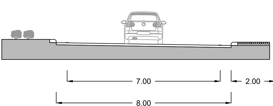
Sezione F-F
