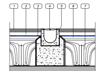
DETTAGLIO CANALETTA DI DRENAGGIO CON CADITOIA LINEARE
