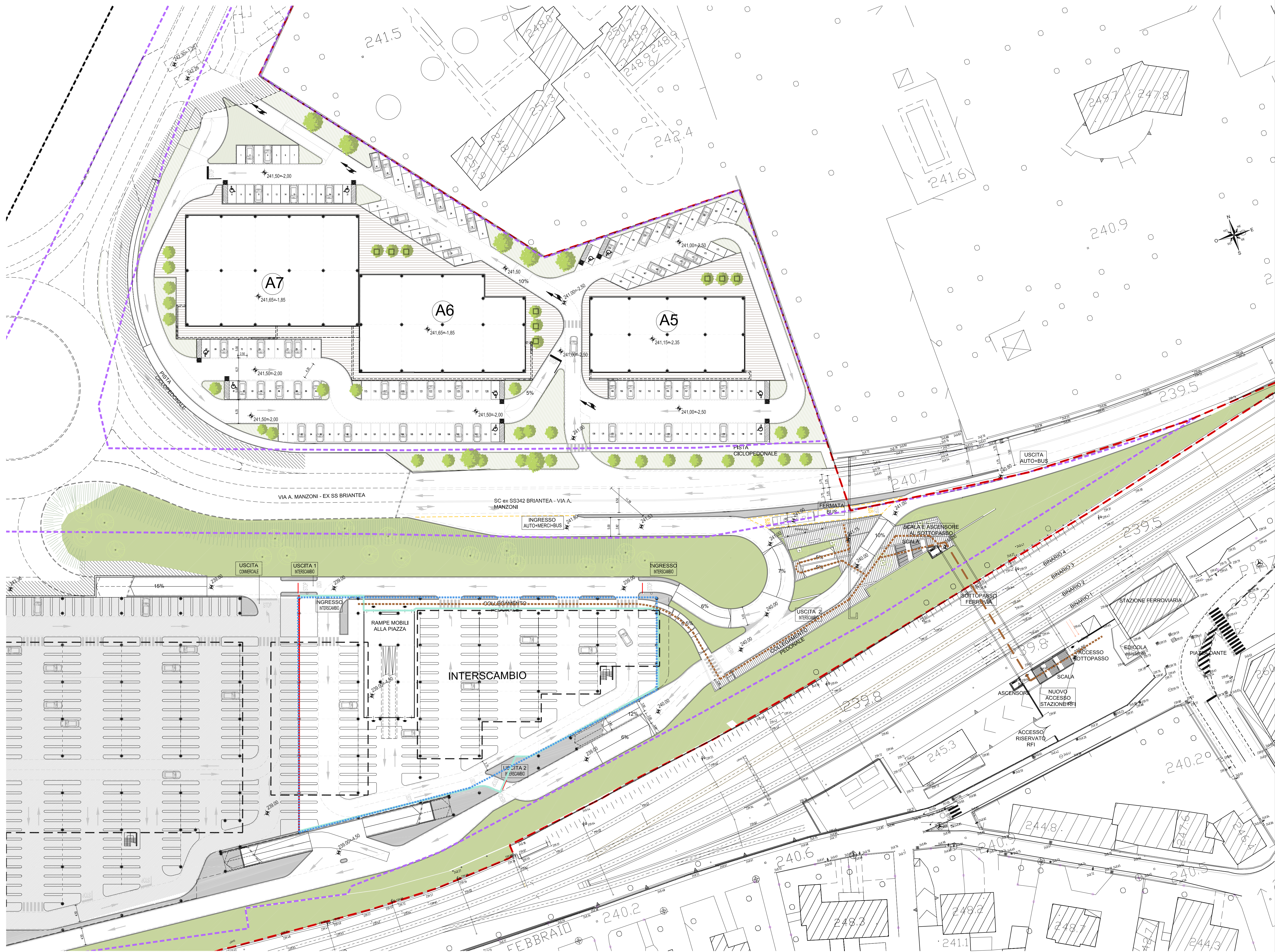
PIANTA - SCALA 1:200
