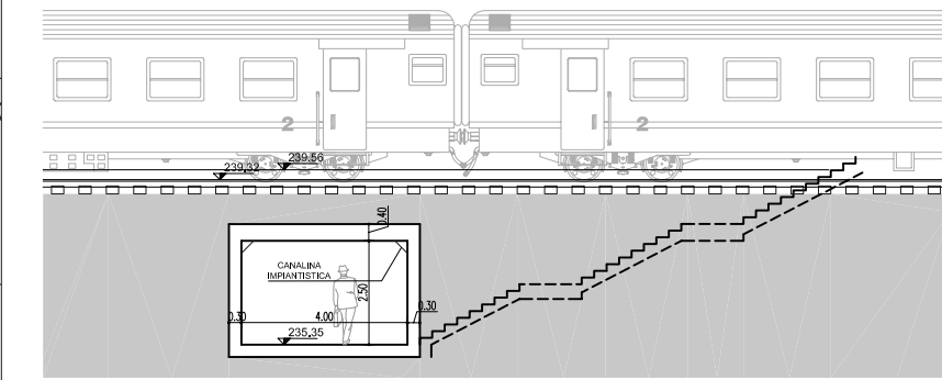
SEZIONE TIPO - SCALA 1:200
