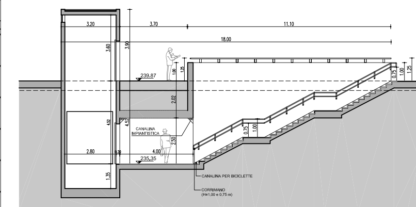
SEZIONE B-B - SCALA 1:200
