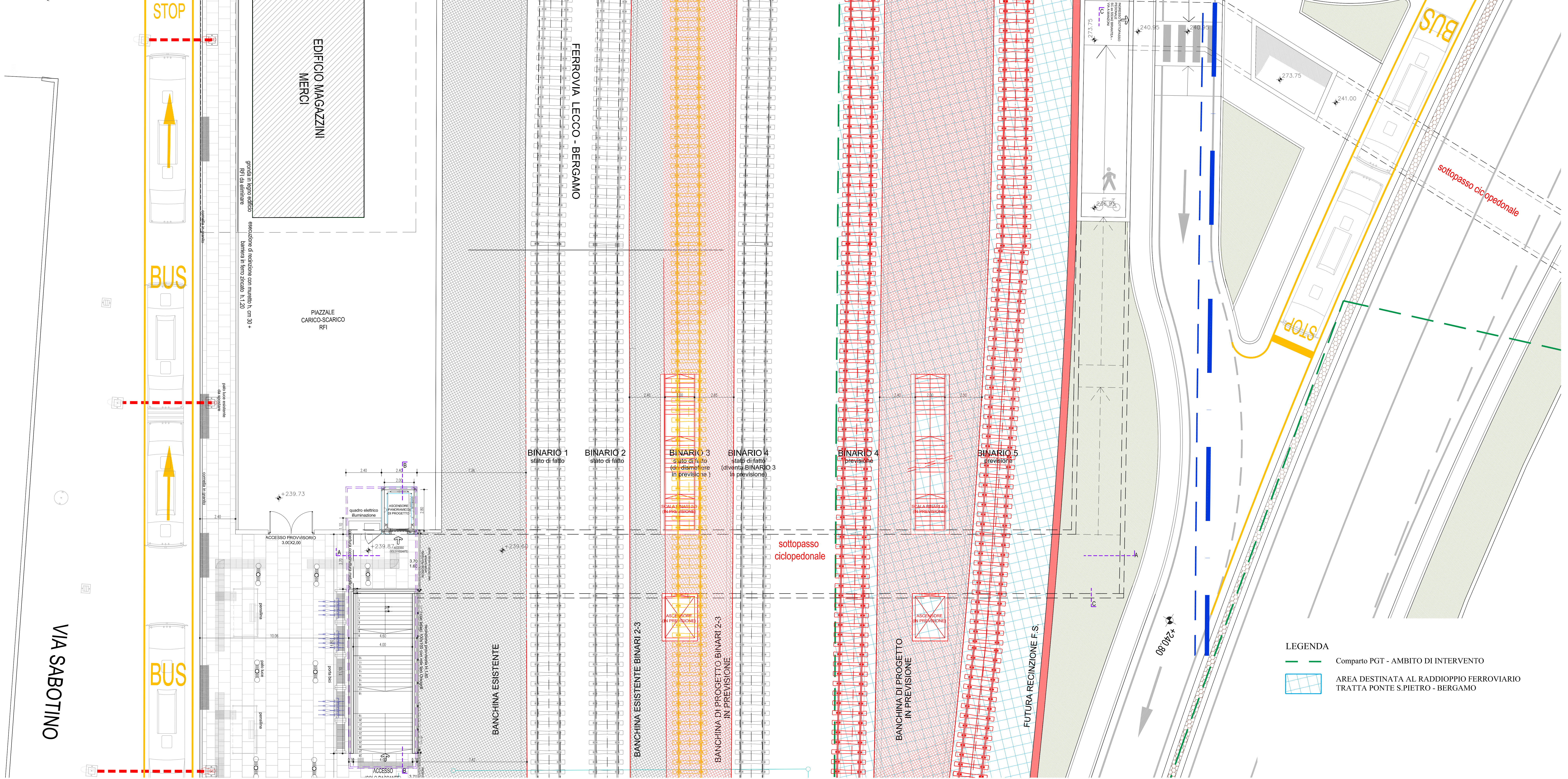
PIANTA SOTTOPASSO
