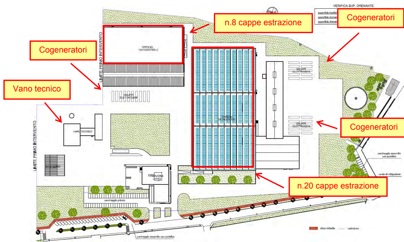
Figura 10 - Stralcio planimetrico progetto Aruba con indicazione degli impianti individuati.
