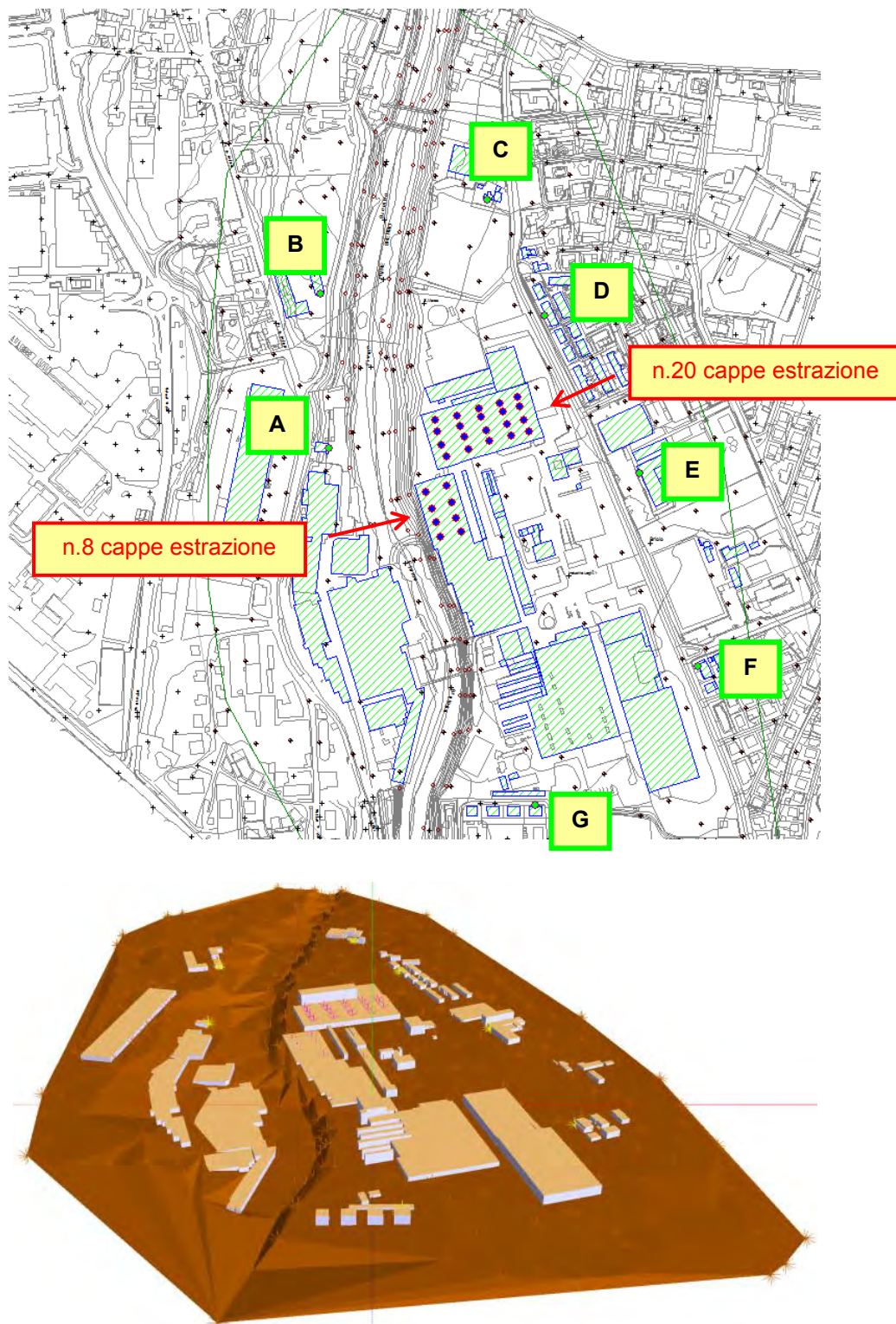
Figura 12 - Stralci SoundPlan 2D e 3D con indicazione delle sorgenti inserite e dei punti di verifica ai recettori.
